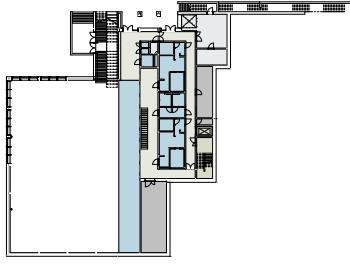
1:500 U1. etasje Kote 40000
